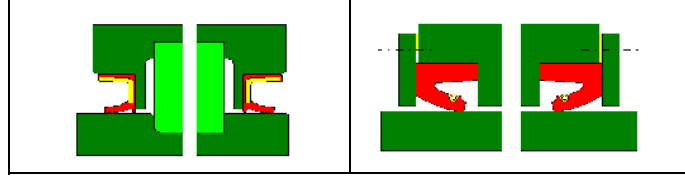
スイングレバー・トラニオン軸受
