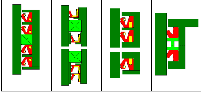
回転分級機・ロータリーセパレーター
