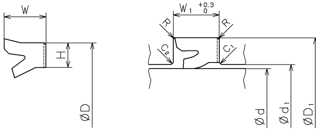
シール断面
